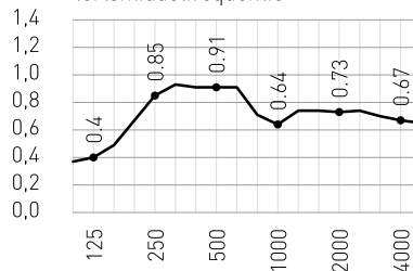
geluidsabsorptiegraad tot tertsmiddelfrequentie
